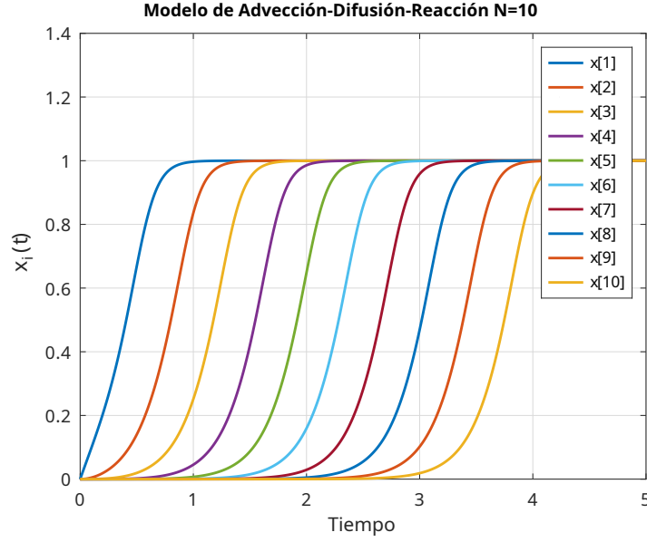
(a) Solución numérica del sistema ADR con N = 10
