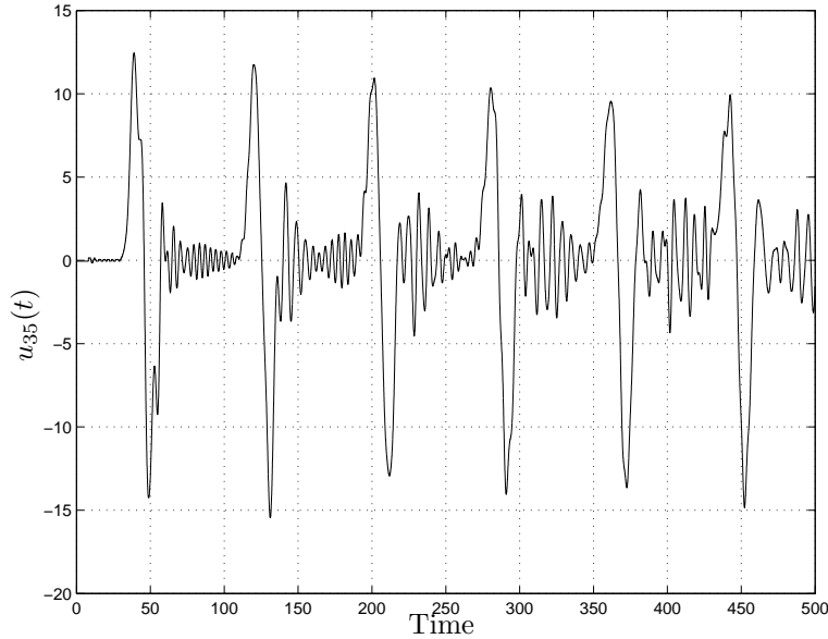
Figura 4.12: Simulación con CQSS del sistema representado por (4.47)–(4.49)
