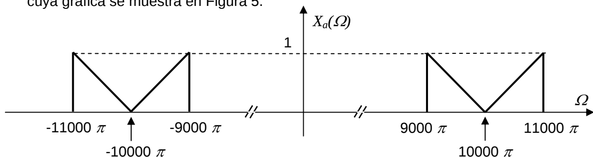
Figura 5: Espectro X_a(\Omega) (no periódico).
