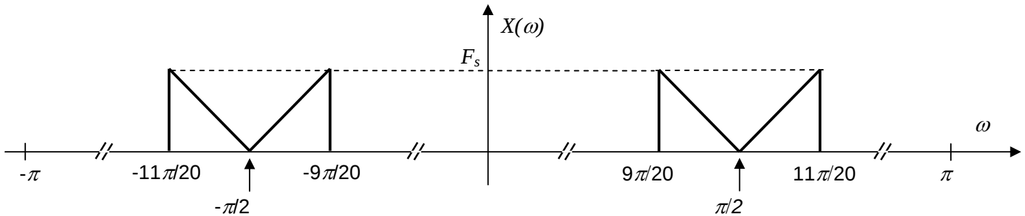
Figura 6: Espectro X(\omega) ( periódico, con período 2\pi en \omega ).
