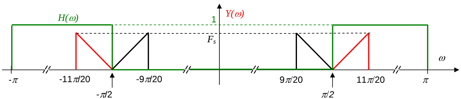
Figura 7: Espectro Y(\omega) ( periódico, con período 2\pi en \omega ).
