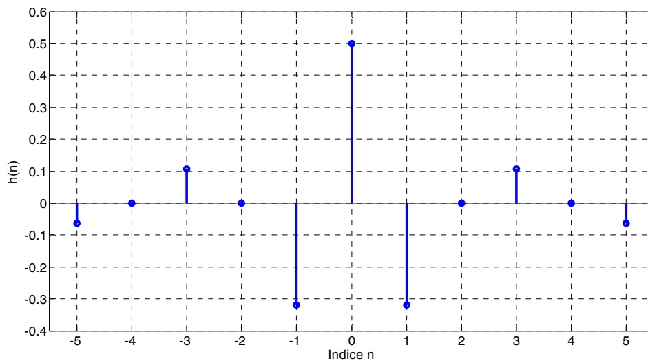
Figura 3: Respuesta al impulso del filtro pasa altos.
