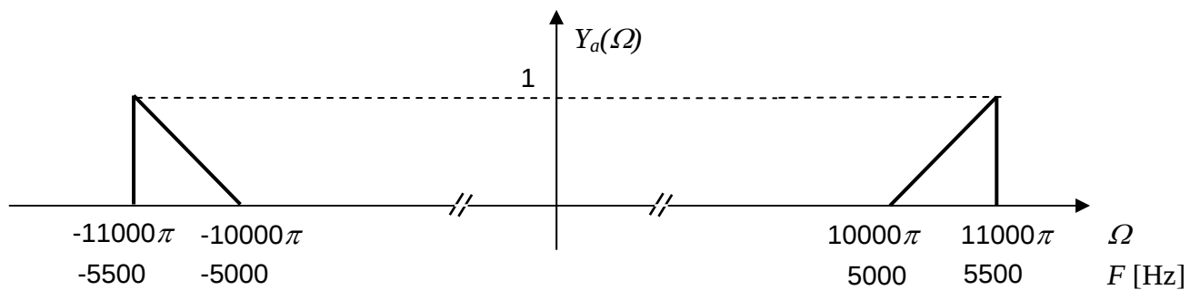
Figura 8: Espectro Y_a(\Omega) ( no periódico ).
