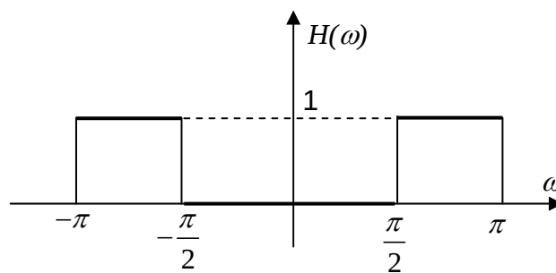
Figura 2: Respuesta en frecuencia del filtro pasa-altos.
