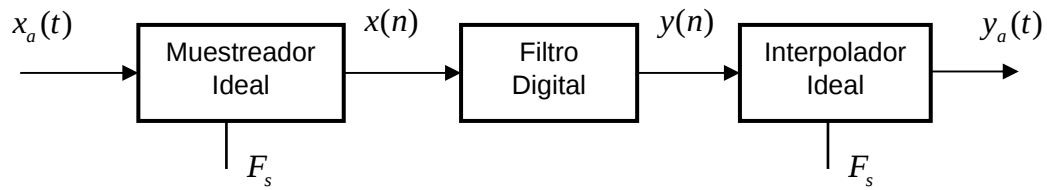
Figura 1: Sistema de Procesamiento Digital de Señales
