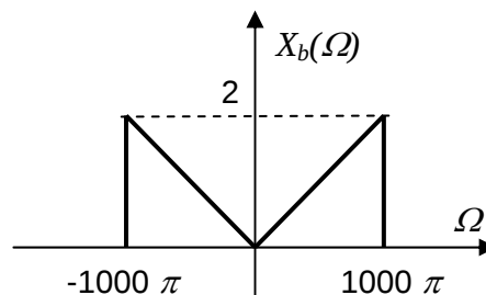
Figura 4: Espectro X_b(\Omega) .
