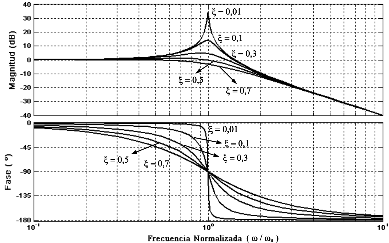
Diagrama de Bode de Sistema de Segundo Orden
