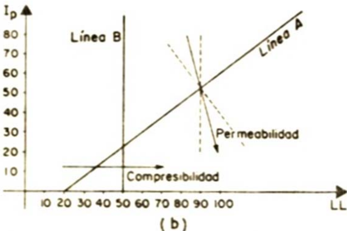
FIG. VII - 3. DIRECCIÓN DE VARIACIÓN DE ALGUNAS PROPIEDADES FÍSICAS DE LOS SUELOS EN LA CARTA DE PLASTICIDAD.
