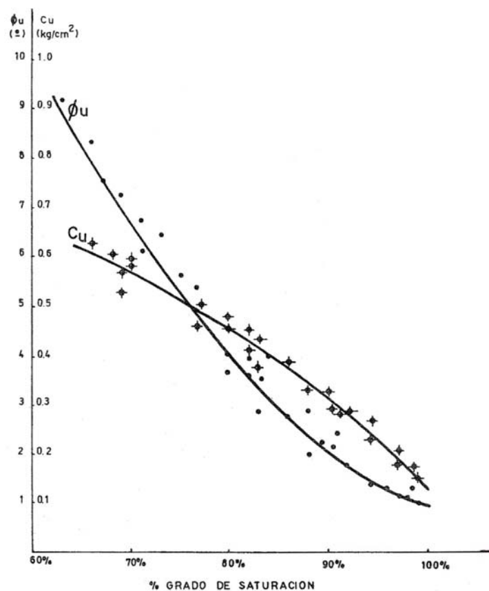
Figura 5: Variación de los parámetros de ensayos triaxiales no consolidados no drenados con el grado de saturación. 1 kg/cm 2 = 98.1 KN/m 2 (Núñez et al., 1970).
