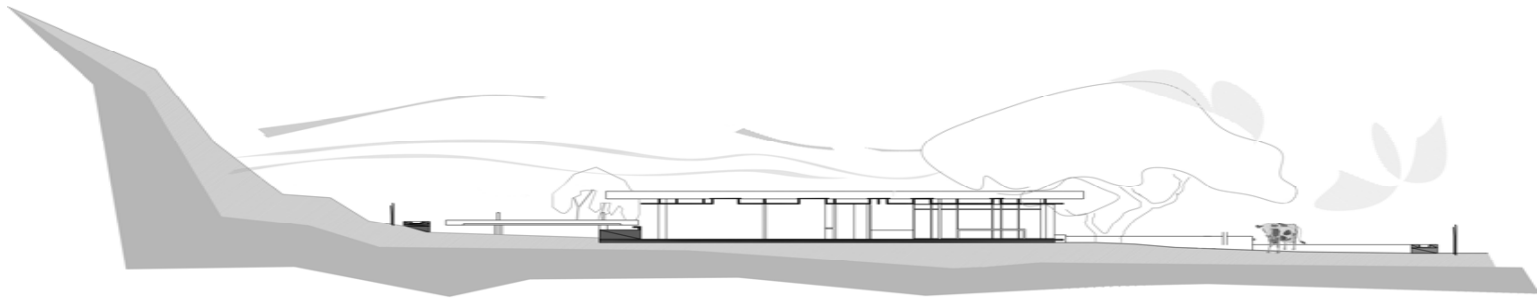
CORTE D-D
