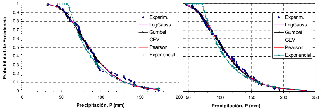
Figura 2.- Probabilidad de excedencia, luvias de D=1 día (izquierda) y D=2 días (derecha), Rosario.
