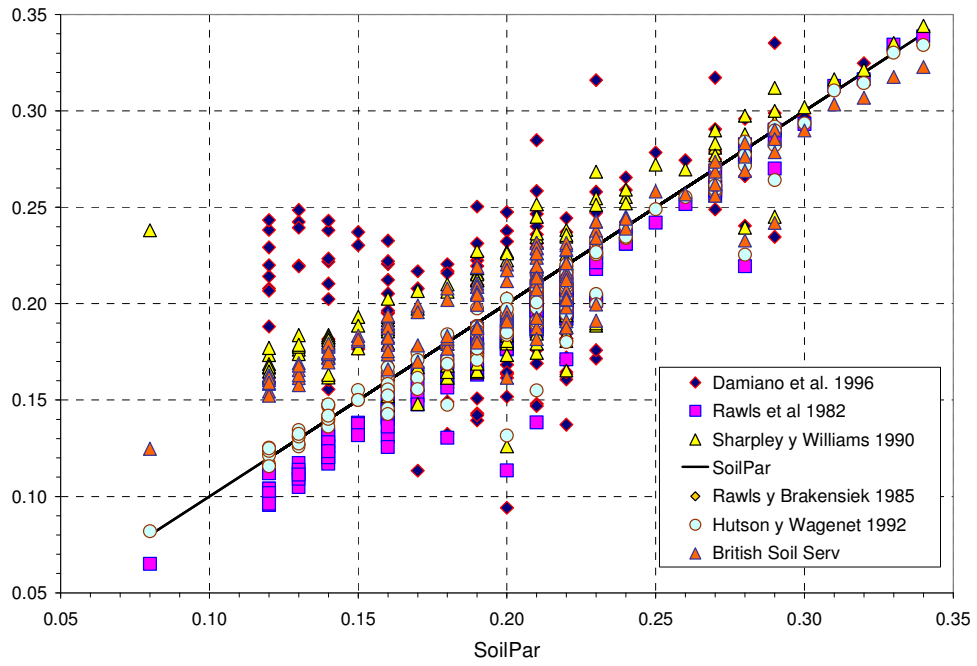
Figura 3. Estimación del punto de marchitez permanente, \theta_{-1500}
