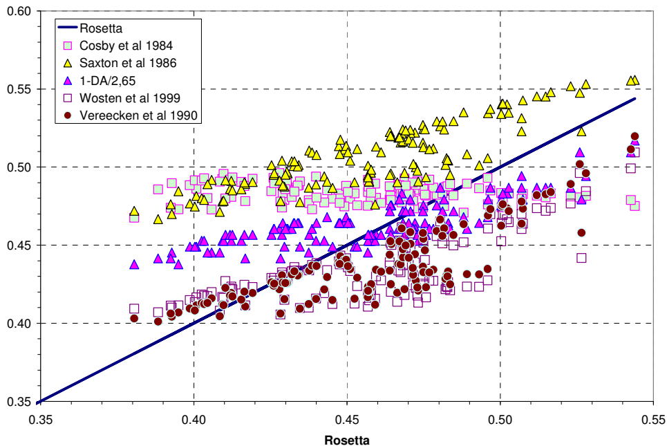
Figura 5. Estimación de la humedad de saturación, \theta_s
