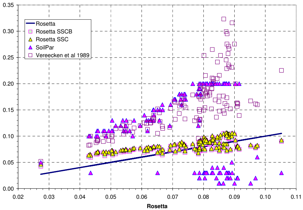
Figura 4. Estimación de la humedad residual, \theta_r
