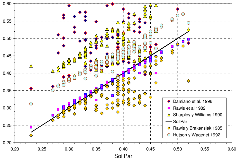
Figura 2. Estimación de la humedad de capacidad de campo, \theta_{33}
