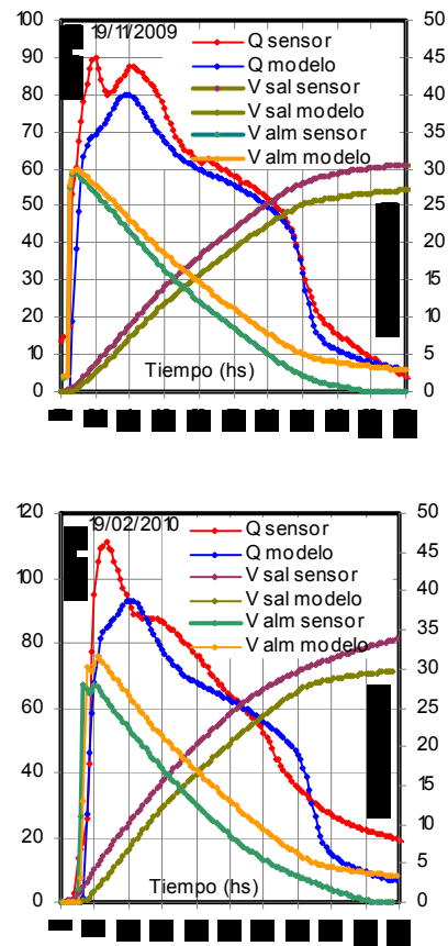
Fig. 4. Caudales y volúmenes salientes y almacenados
