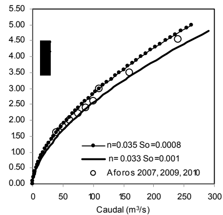
Fig.2. Curva H-Q sitio Circunvalación
