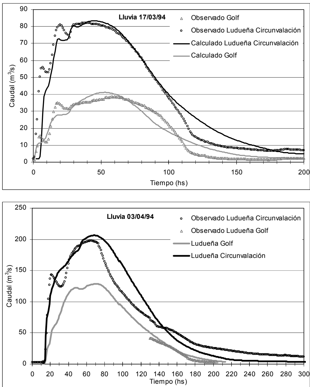
Figura 3. Hidrogramas Observados y Calculados
