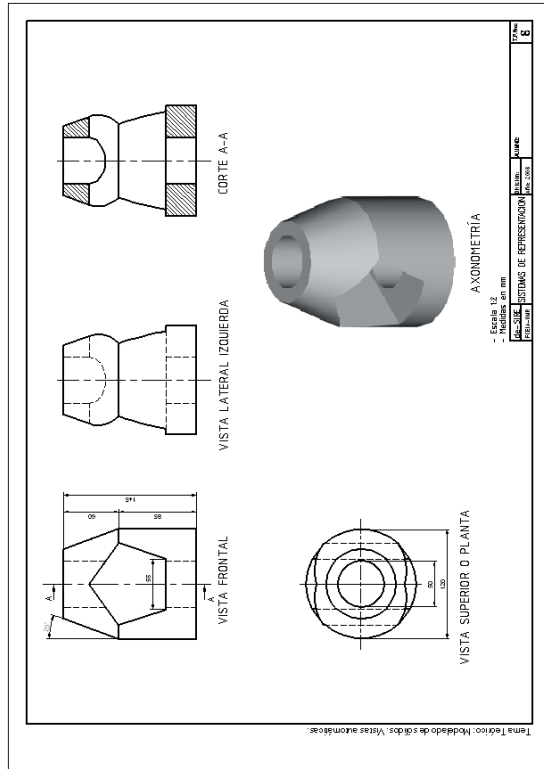
Figura 11. Plano de definición a presentar por los alumnos.
