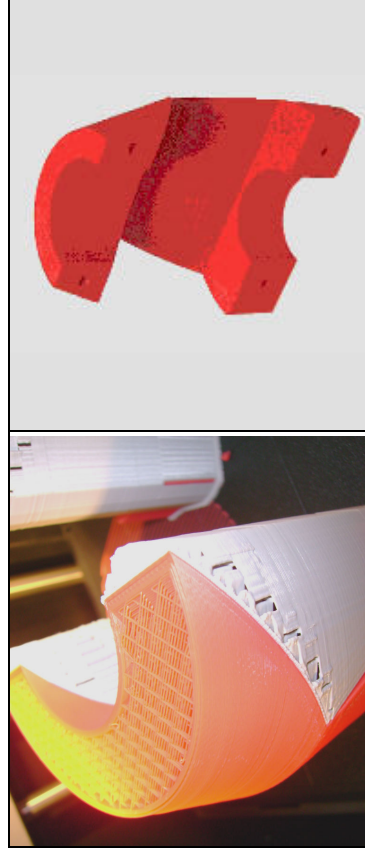
Figura 7. Detalle entramado interno y material de soporte. Prototipo hembra con cavidades para encastre de tetones.
