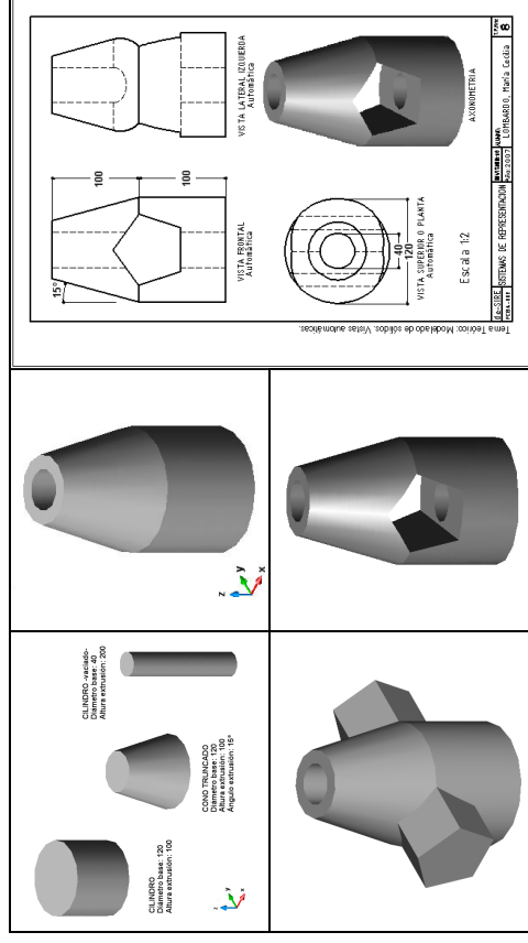
Figura 5. Tutorial del proceso de modelado sólido 3D. Vistas automáticas y axonométrica presentadas por un alumno.
