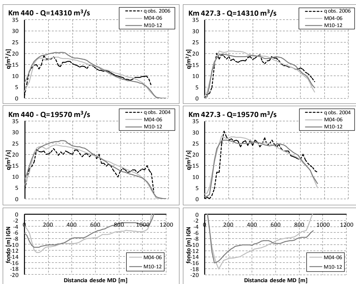
Figura 7.- Comparación de la distribución de caudales unitarios q calculados y observados (FICH,2006) y nivel del fondo del MDT (a) Sección transversal km 440 (b) Sección transversal km 427.3.
